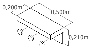
Estantes
