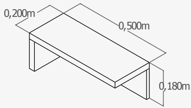
Estante colgador 50
