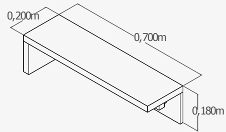
Estante colgador 70
