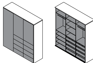
3A8 210x60x230 3 cossos; portes abatibles; 8 calaixos
