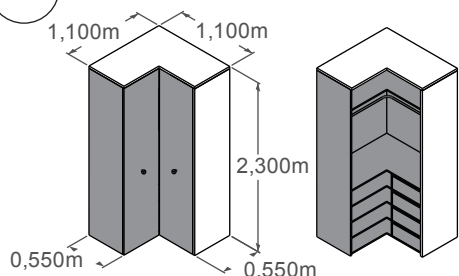
2A4L 110x110x230 2 cossos; portes abatibles; 4 calaixos; forma L
